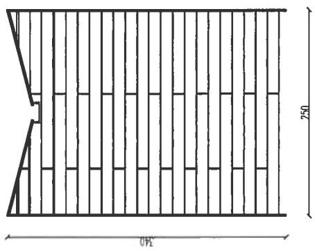
PROSPETTO TIPO LATO CORTO
